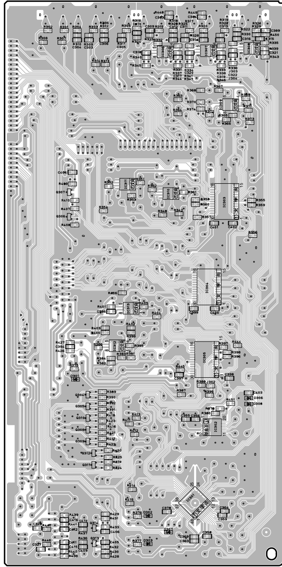
FUNCTION (6) CB401
